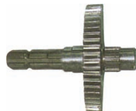
ANH-835 PTO SHAFT (6/55/25 T) 5630
